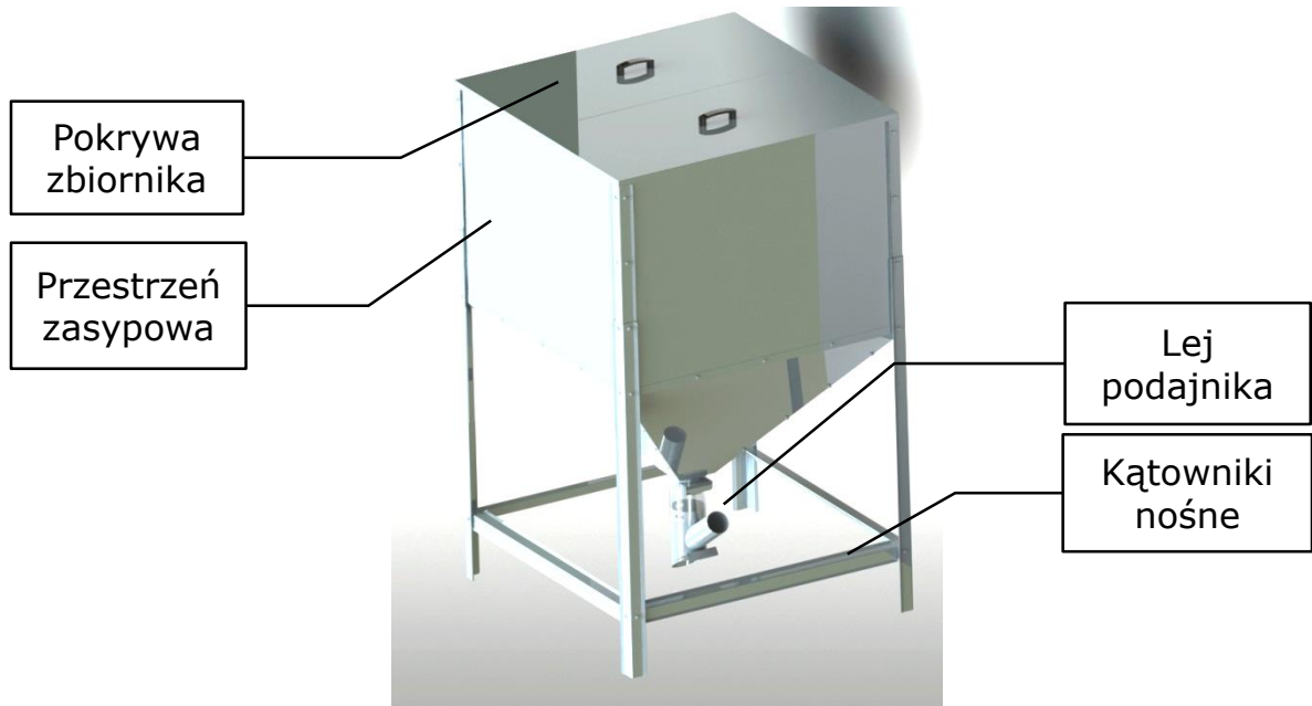
Rys. 1. Budowa zbiornika.
