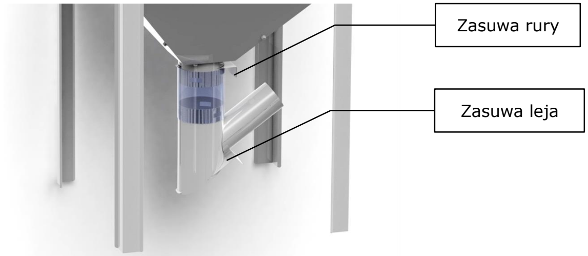
Rys. 6. Pozycja zasuwek.
