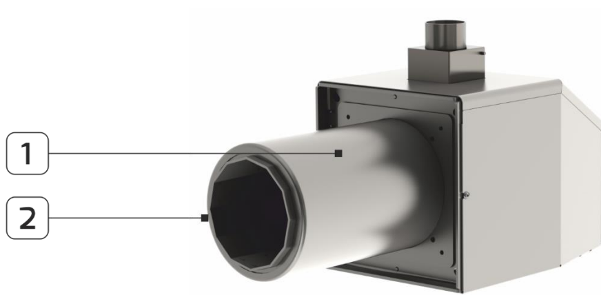
Rys. 11. Konserwacja palników od REVO 44 do REVO 150.
