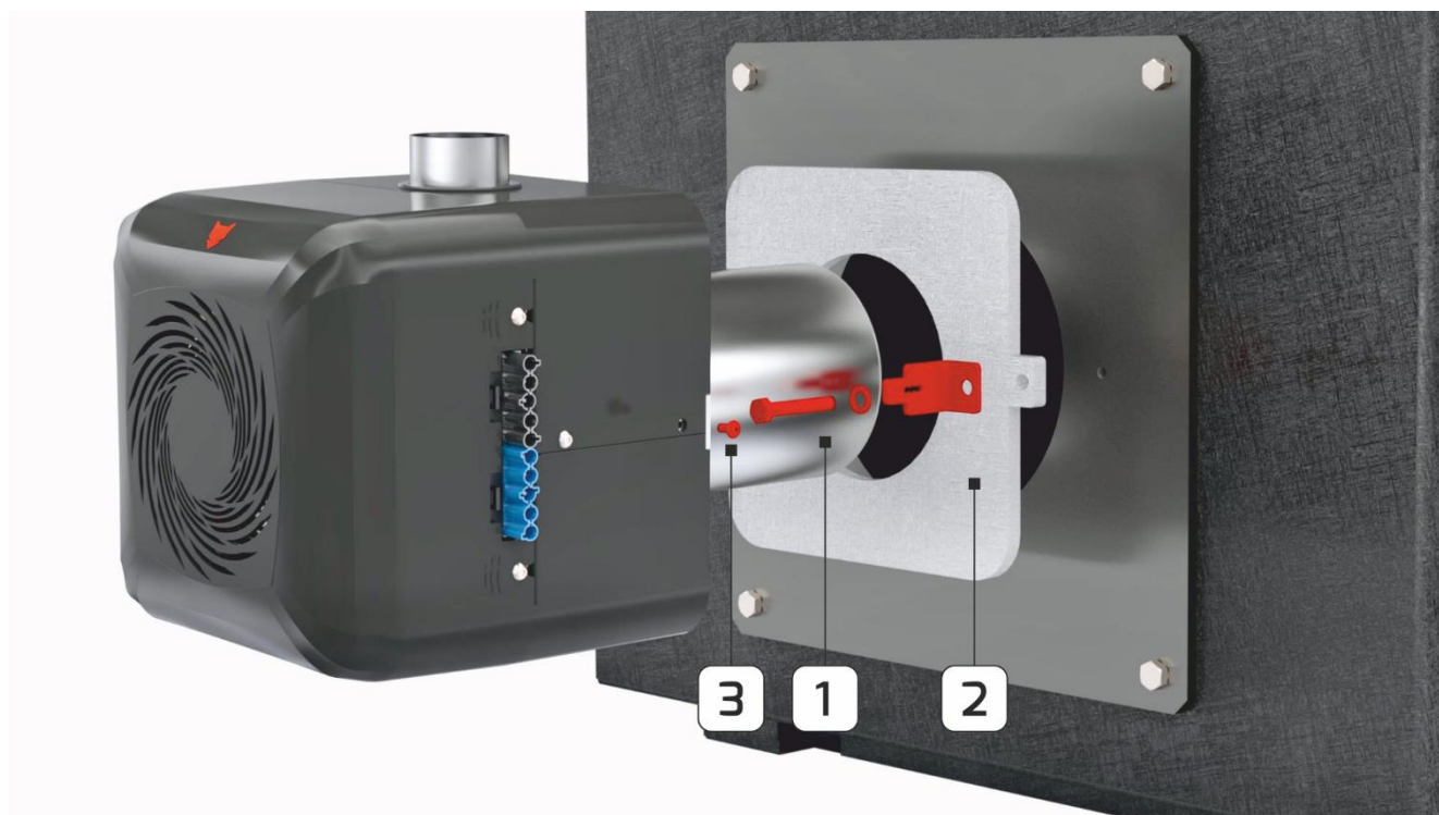
Rys. 8. Montaż modeli palników REVO Micro 16, Mini 26 i Mini 35 w drzwiach kotła.
