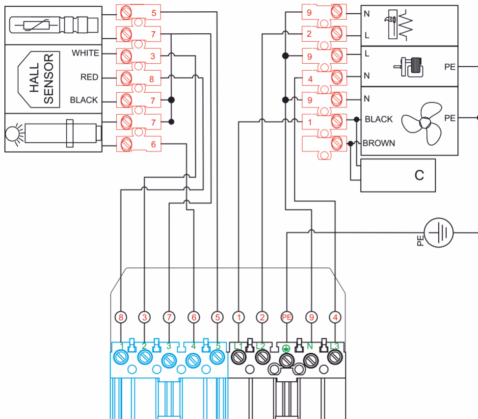
Rys. 14. Schemat elektryczny modeli REVO Mini 26 i Mini 35.
