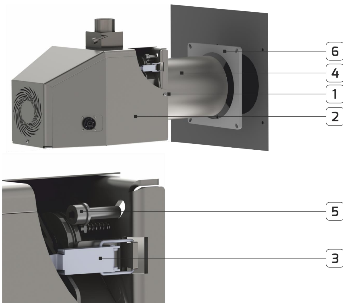
Rys. 9 Montaż modeli palników od REVO 44 do REVO 150 w drzwiczkach kotła.
