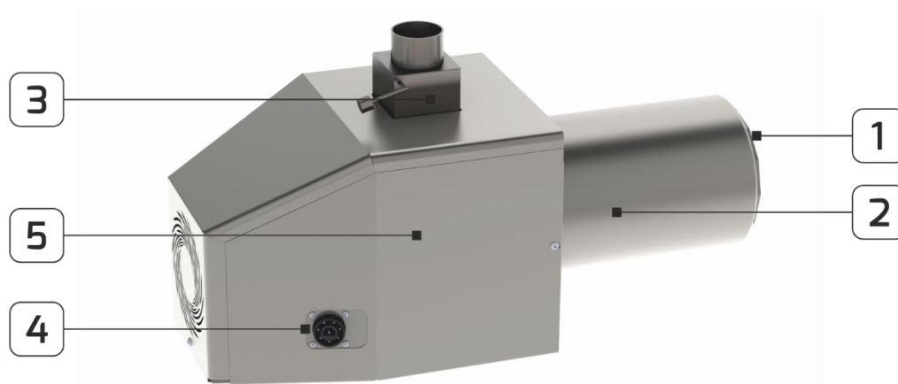
Rys. 2. Budowa palnika od REVO 44 do REVO 150.
