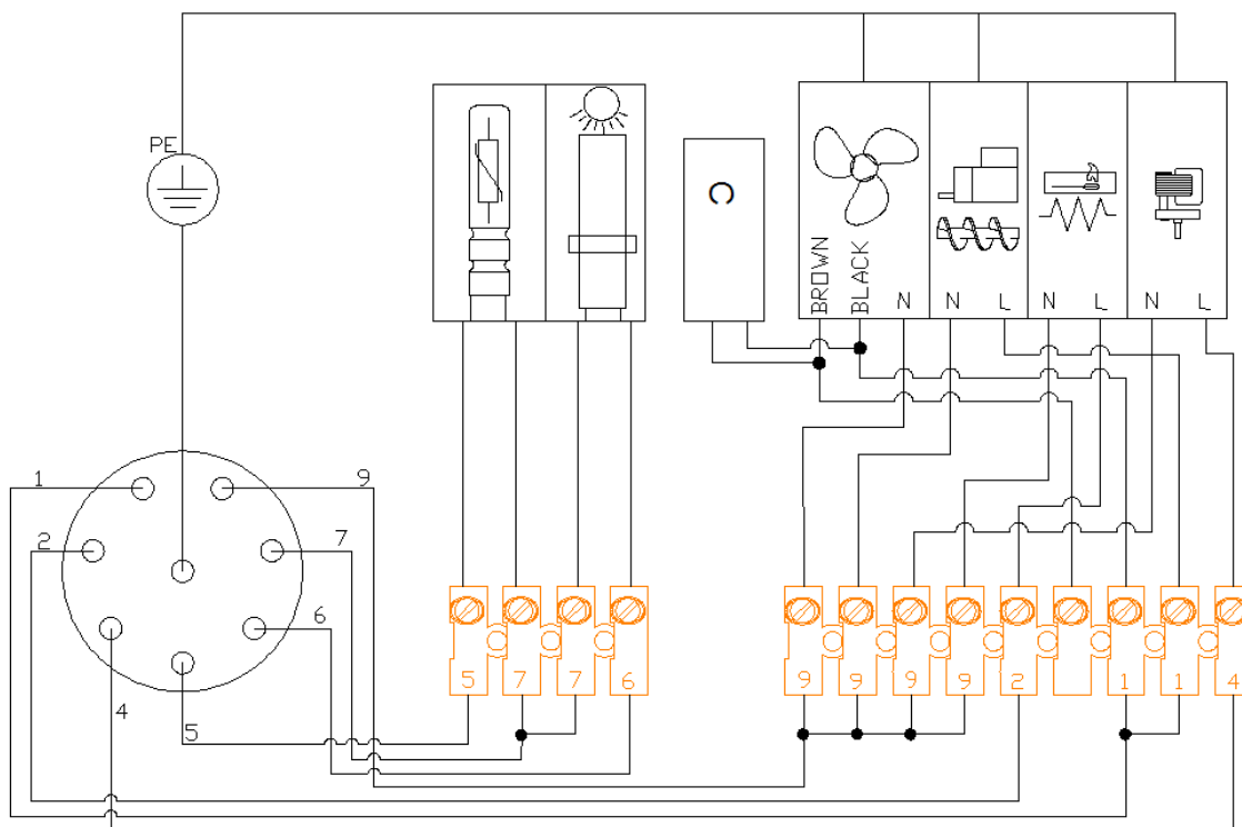
Rys. 15. Schemat elektryczny modeli od REVO 44 do REVO 150.
