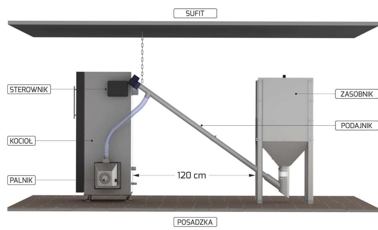
Rys. 7. Schemat instalacji kotłowni.
