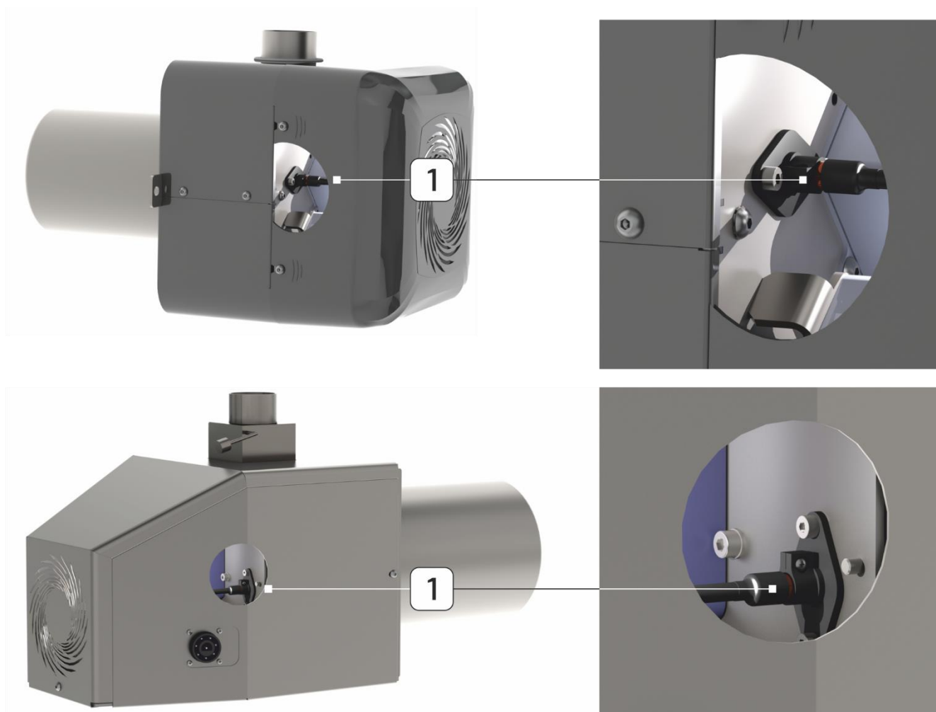
Rys. 12. Pozycja fotosensora w palnikach REVO.
