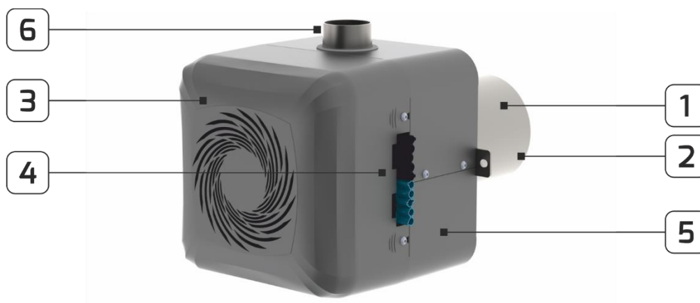
Rys. 1. Budowa palnika od REVO Micro 16 do REVO Mini 35.
